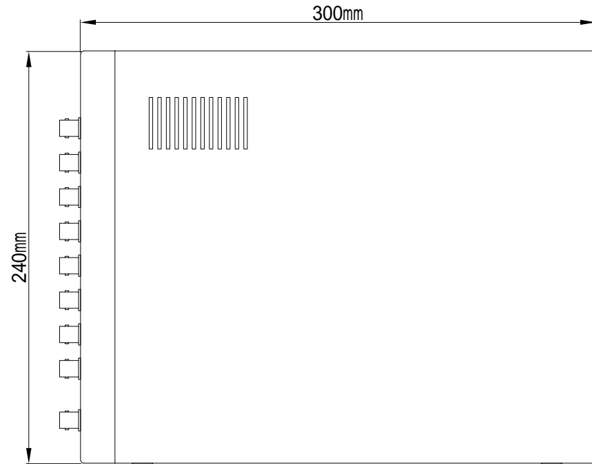
A/DコンバータBOX(例：16ch)
