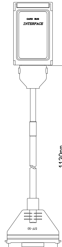
I/Fケーブル
