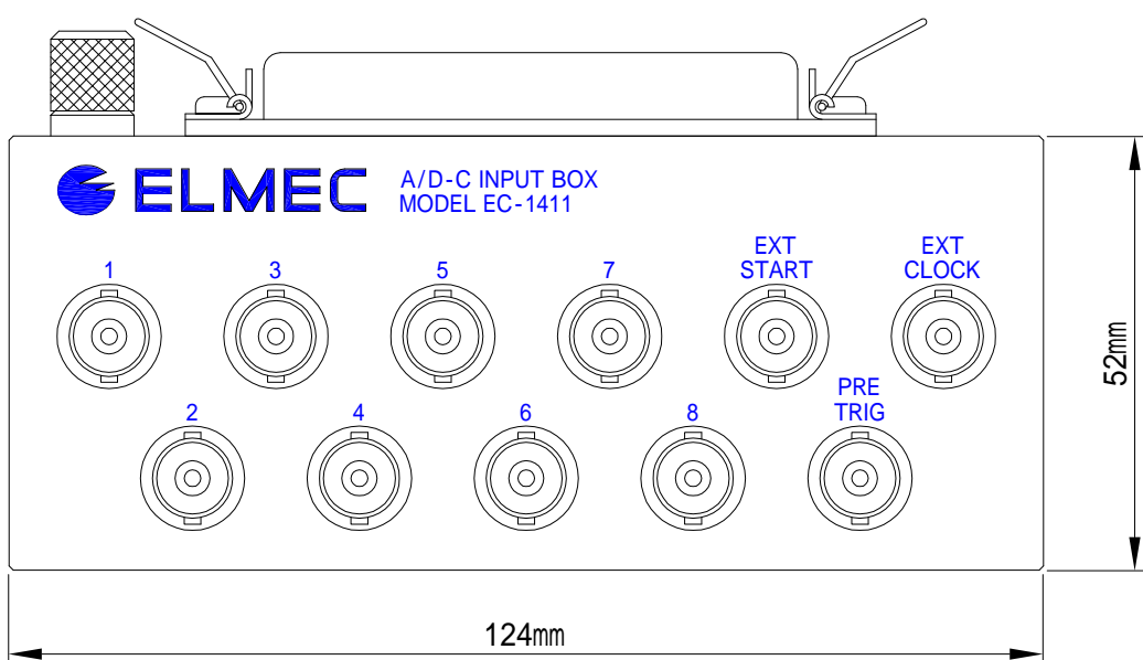
EC-1411D(差動入力タイプ)
